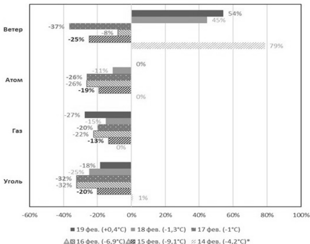
Рис. 7 / Fig. 7. Сравнение изменения электрогенерации в условиях аномально холодных температур относительно нормальных температур по типу топлива / Comparison of changes in power generation in conditions of abnormally cold weather relative to normal temperatures by type of fuel
